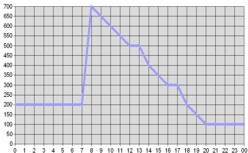
График расхода топлива за сутки
